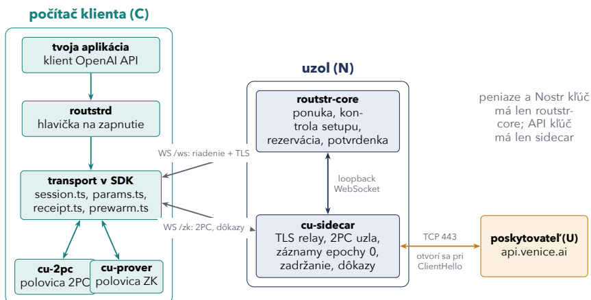
Obr. 6.1: Procesy a kanály. routstr-core kopíruje bajty 2PC a dôkazov bez zmeny; zachytáva len niekoľko riadiacich rámcov.
