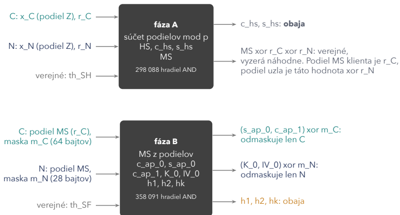
Obr. 8.2: Dva obvody. Tyrkysové vstupy pochádzajú od C, tmavomodré od N, sivé sú verejné; výstupy sú zafarbené podľa toho, kto ich môže čítať.
