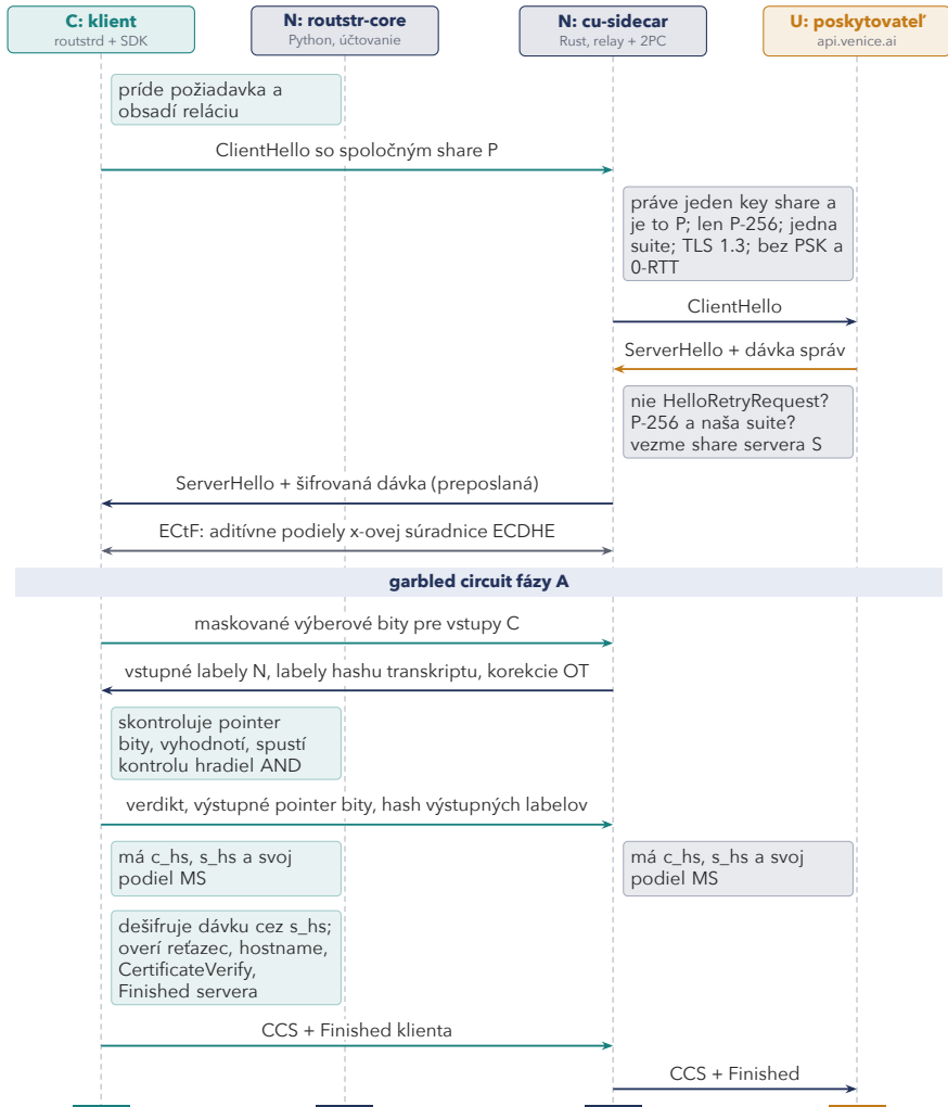
Obr. 7.4: Handshake. Sidecar prepošle ClientHello, len ak jeho jediný key share je spoločný bod.
