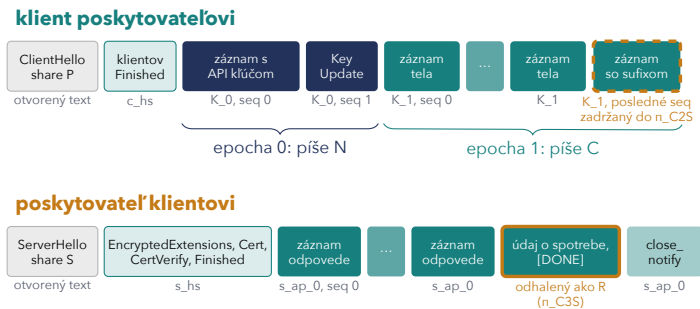
Obr. 4.1: Záznamy jednej relácie tak, ako ich vidí U. Uzol zapíše iba dva tmavomodré záznamy.
