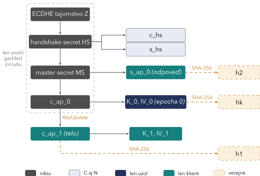
Obr. 3.1: Odvodzovanie kľúčov v TLS 1.3, farebne podľa toho, kto napokon drží ktoré tajomstvo.
