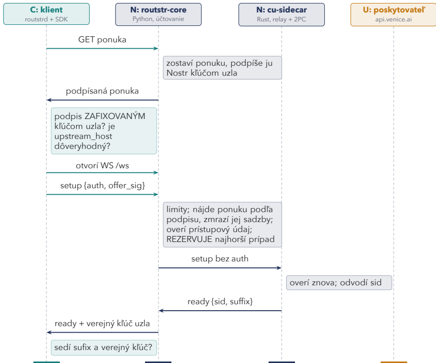
Obr. 7.1: Setup: kým neprejde kontrola prístupového údajá, nič sa nerezervuje, a sidecar prístupový údaj nikdy nevidí.
