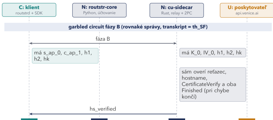
Obr. 7.5: Fáza B dá každej strane jej vlastné aplikačné kľúče; potom sidecar celý handshake overí sám.
