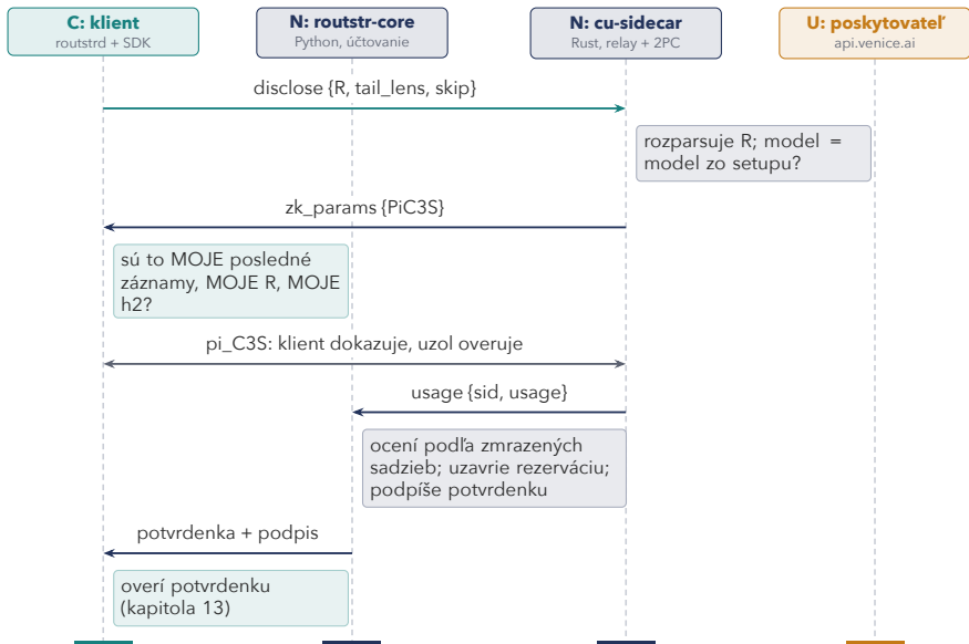
Obr. 7.9: Odhalenie, dôkaz o spotrebe a vyúčtovanie.
