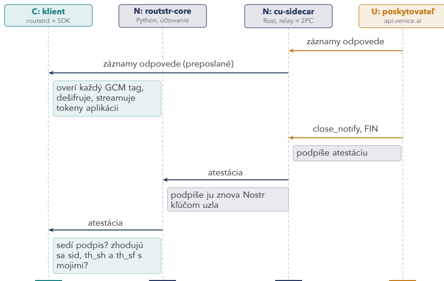
Obr. 7.8: Odpoveď prúdi ku klientovi; uzol atestuje, čo preposlal.
