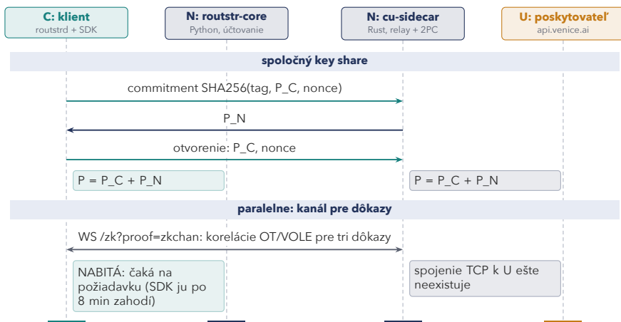
Obr. 7.3: Spoločný key share (najprv commitment, potom otvorenie) a kanál pre dôkazy.
