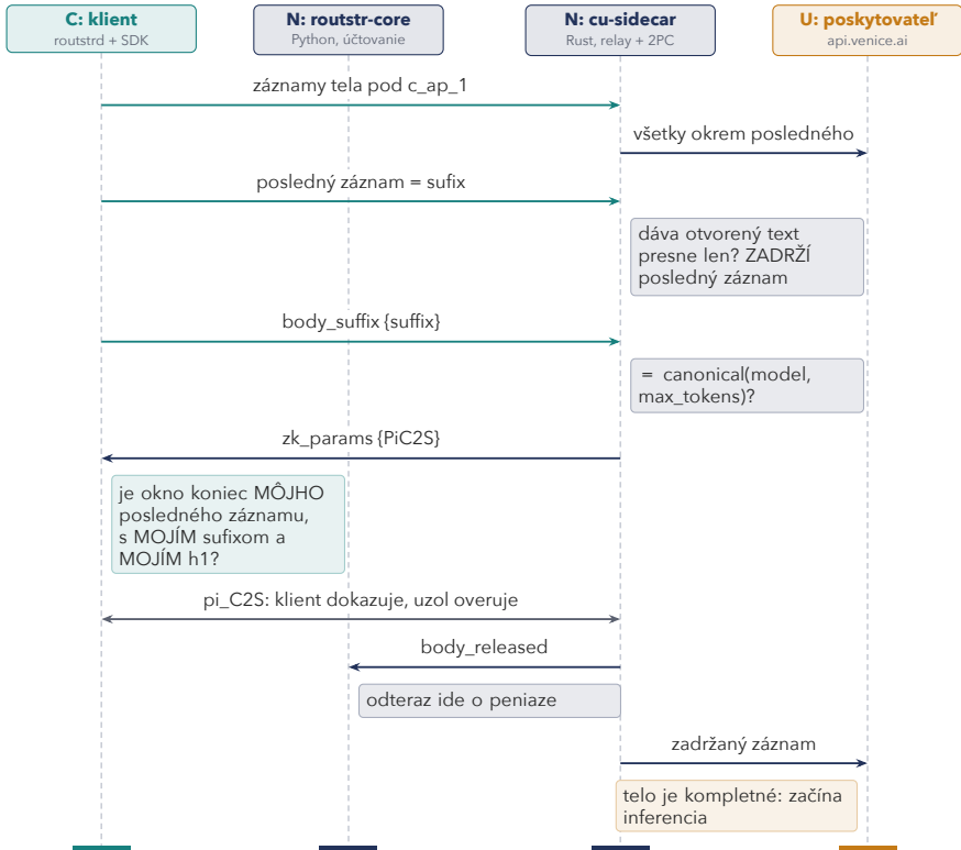
Obr. 7.7: EPOCH 1. Záznam, ktorý dopĺňa telo, zostáva zadržaný, kým neprejde overenie dôkazu o sufixe.
