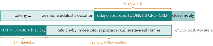
Obr. 9.1: Na čo sa pozerajú n_C2S a n_C3S.
