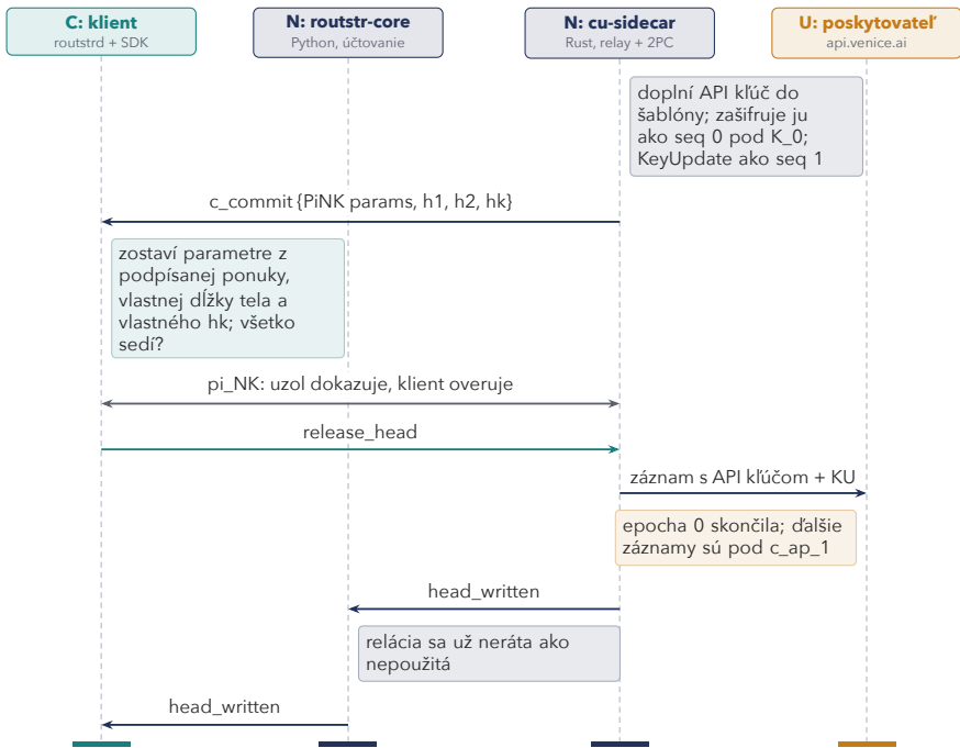
Obr. 7.6: Epocha 0. Uzol sa zaviazal k svojmu záznamu, dokáže, že zodpovedá šablónu, a zapíše ho, až keď klient dá súhlas.
