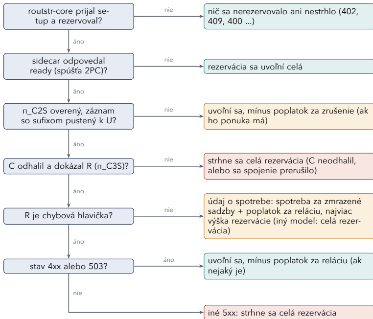
Obr. 12.1: Ako končí rezervácia relácie. Tyrkysová: zadarmo, jantárová: poplatok alebo spotreba, červená: celá rezervácia.
