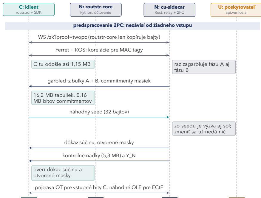
Obr. 7.2: Predspracovanie: drahá časť 2PC, ktorá nezávisí od vstupov. Každý jej bajt môže prebehnúť skôr, než nejaká požiadavka vôbec existuje.
